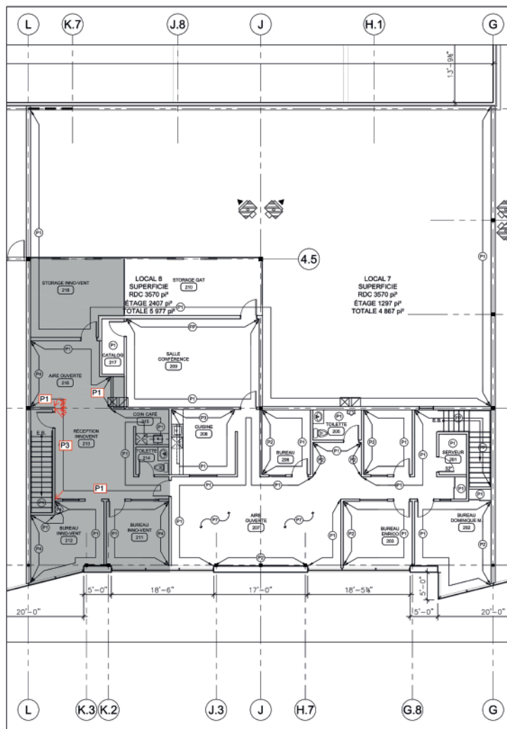
2 PLAN DES PEINTURES DE L'ÉTAGE ÉCHELLE: 1/8"=1'-4"
