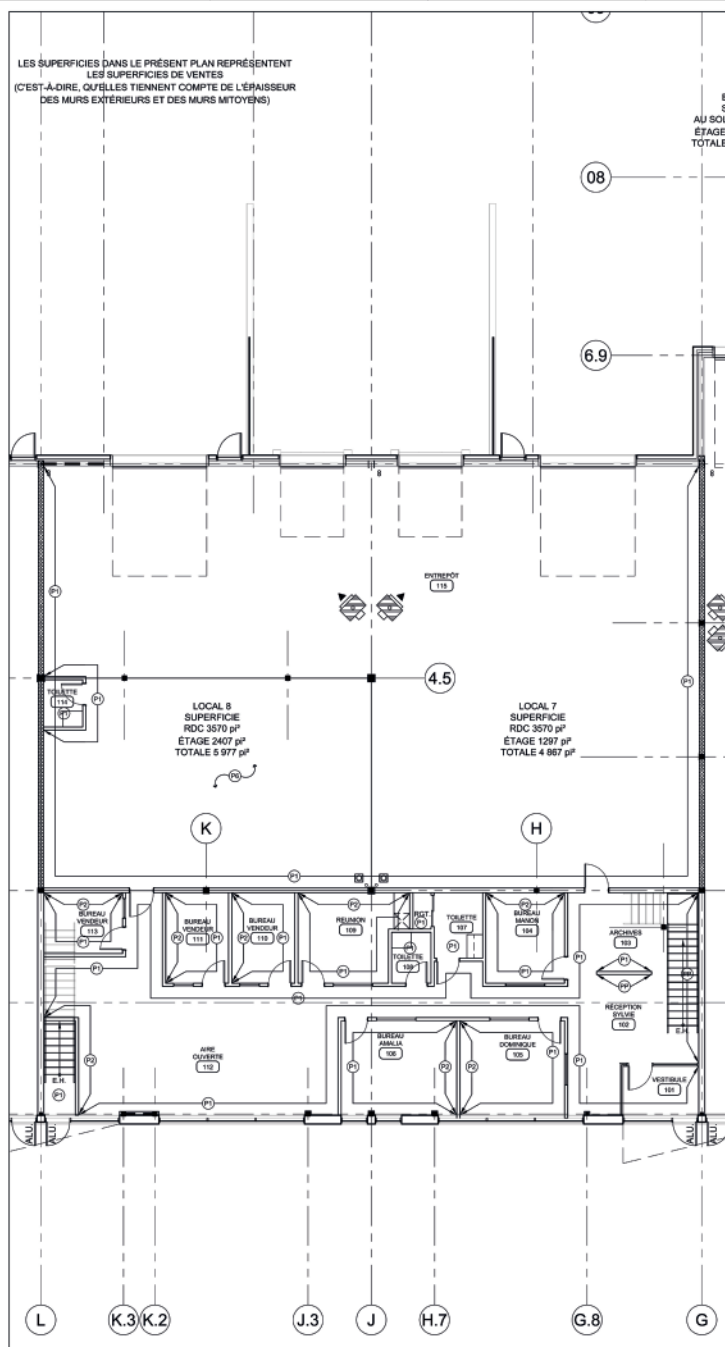
1 PLAN DES PEINTURES DU REZ-DE-CHAUSSÉE ÉCHELLE: 1/8"=1'-4"
