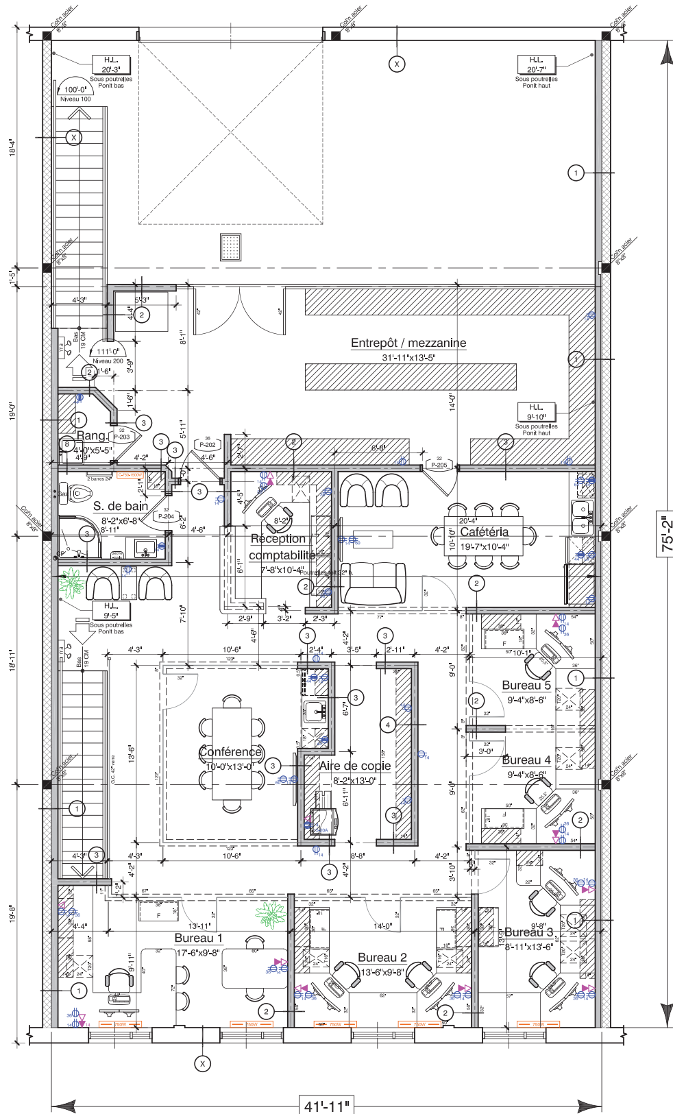
Niveau 200
