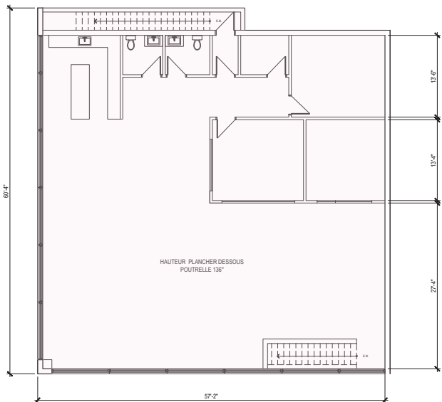
1 PLAN ÉTAGE LOCAL 2 A-100 ECHELLE: 1/8" = 1'-0"
